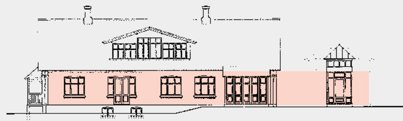
FACADE MOD SYD
